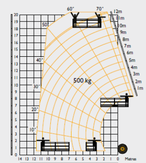
540-200 HiViz Man platform Stabilisers extended
